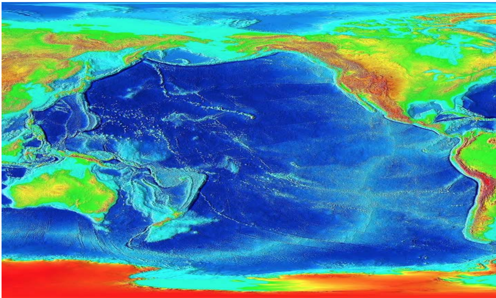
Imagen del fondo del océano Pacífico. Las características más notables son las fosas situadas en el lado occidental y las grandes llanuras que se extienden por el lado oriental.
